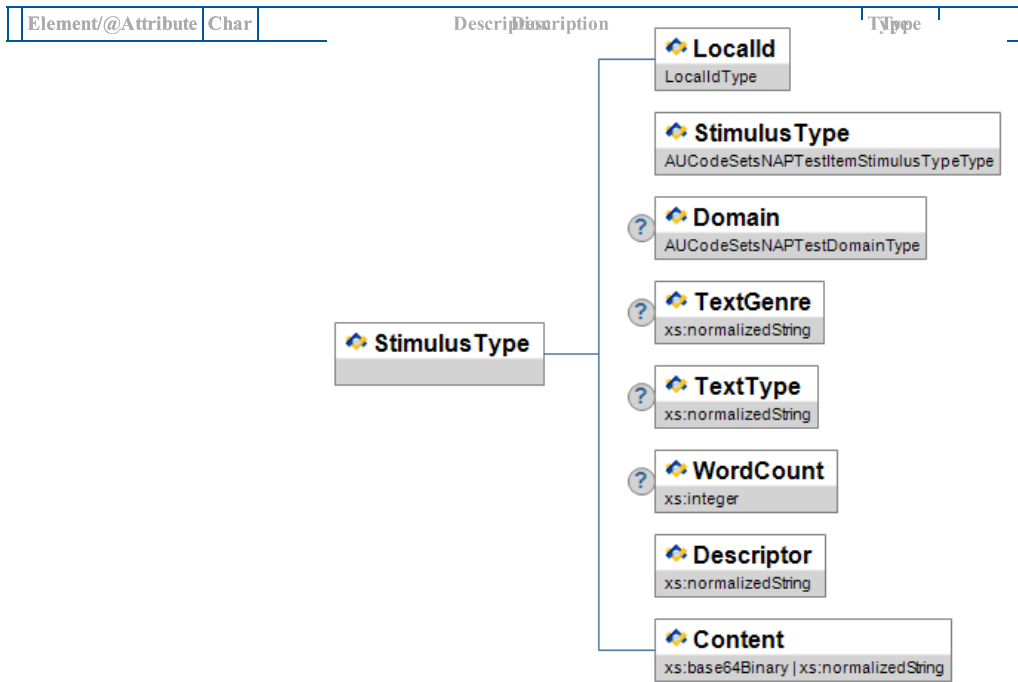
Figure A.162-1: StimulusType
