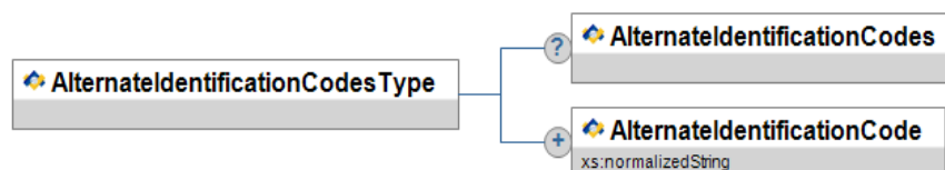
Figure A.14-1: AlternateIdentificationCodesType
